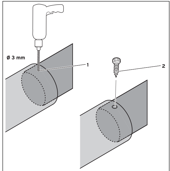
Рис. 4.32 Фиксация телескопических удлинителей
