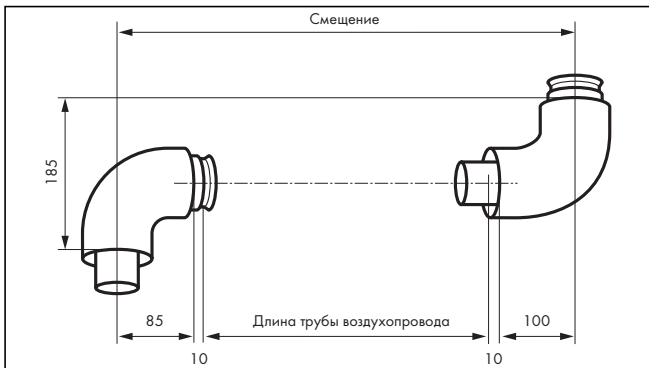
Рис. 4.29 Монтаж колен 90°
