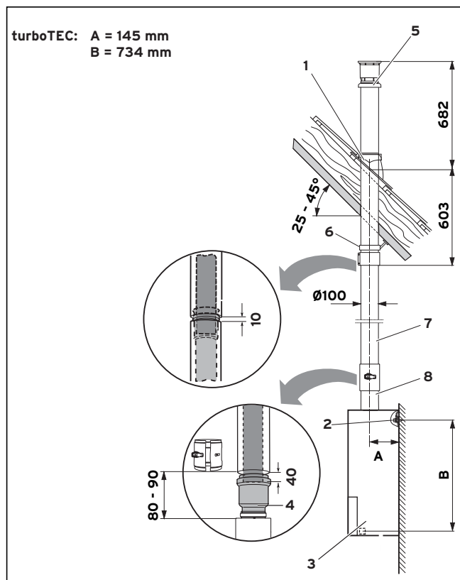
Рис. 4.17 Монтаж прибора и кровельного ввода
