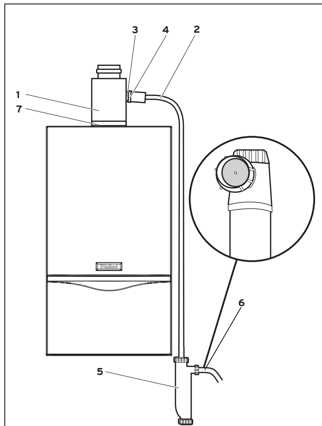
Рис. 4.15 Монтаж соединителя прибора
