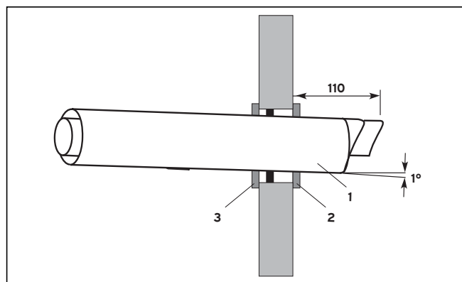
Рис. 4.21 Вмонтаживание горизонтального кровельного ввода
