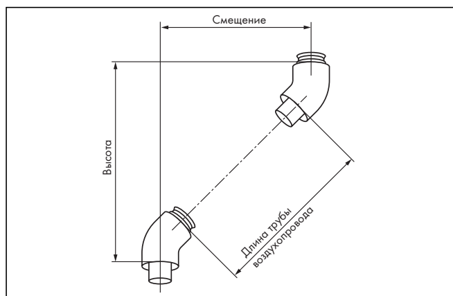
Рис. 5.29 Монтаж колен 45°
