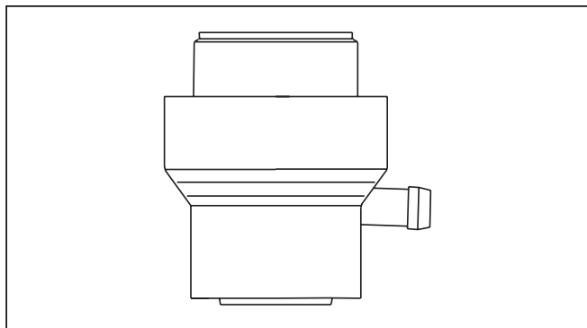
Рис. 5.1 Соединитель прибора, Ø 80/125
