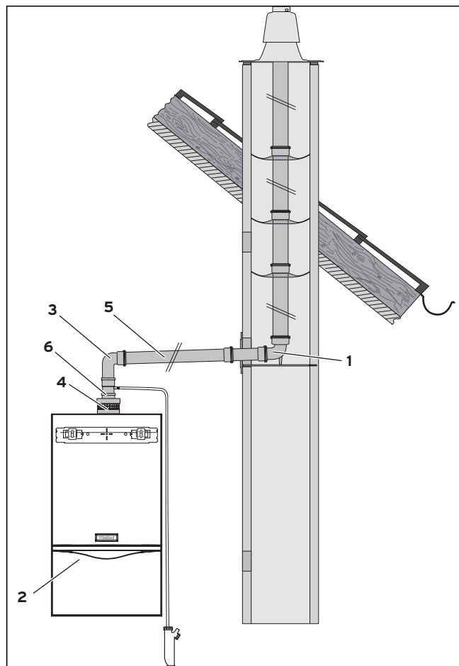
Рис. 6.11 Монтаж
