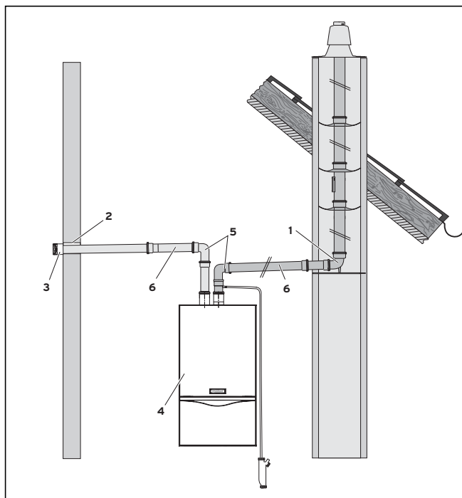
Рис. 6.17 Поддача дутьевого воздуха через наружную стену
