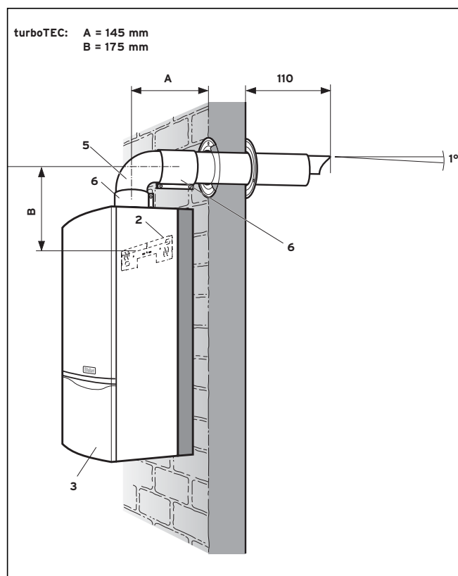
Рис. 4.25 Монтаж прибора (прямая установка)
