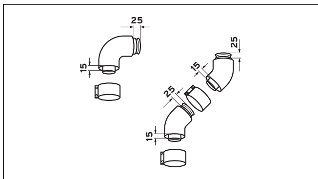
Рис. 5.3 Колена, Ø 80/125
