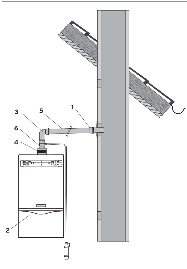
Рис. 6.12 Монтаж
