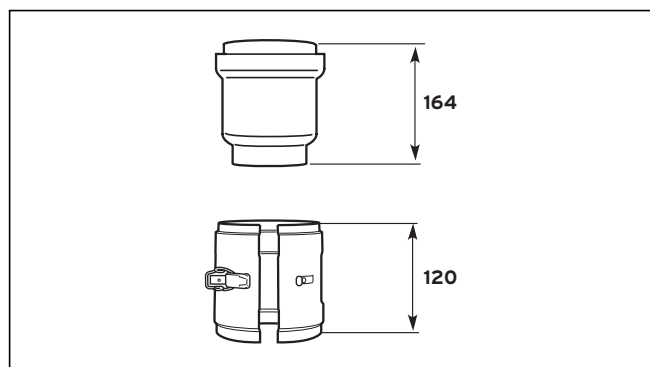
Рис. 5.5 Разделитель, Ø 80/125
