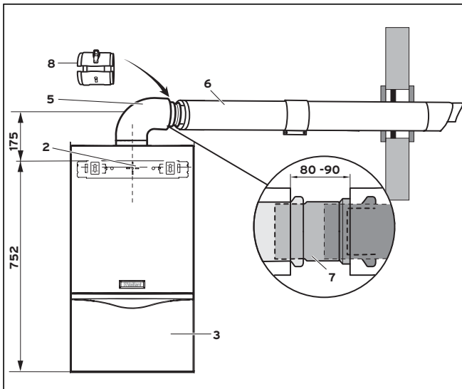
Рис. 4.26 Удаленная установка
