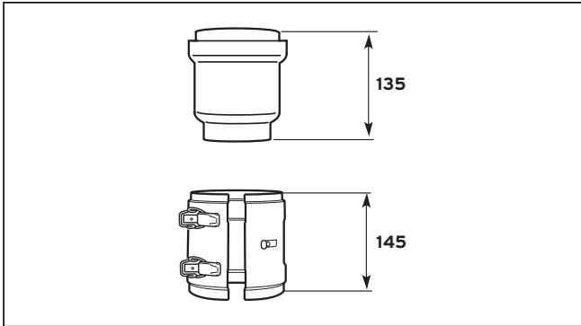
Рис. 4.7 Разделитель, Ø 60/100
