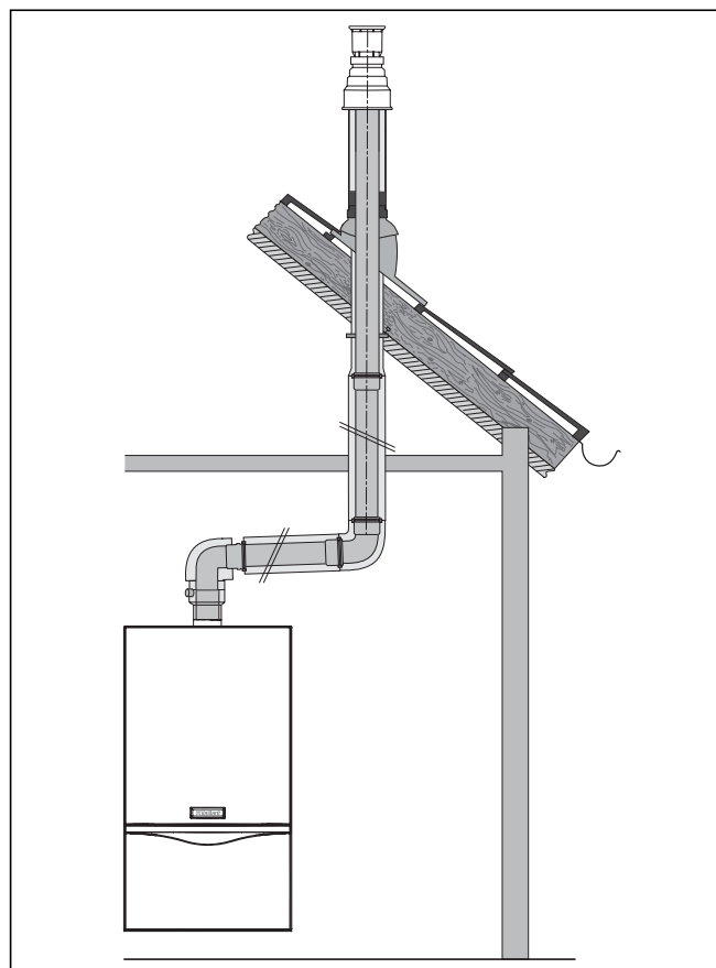
Рис. 5.18 Пример монтажа вертикального кровельного ввода с отводом
