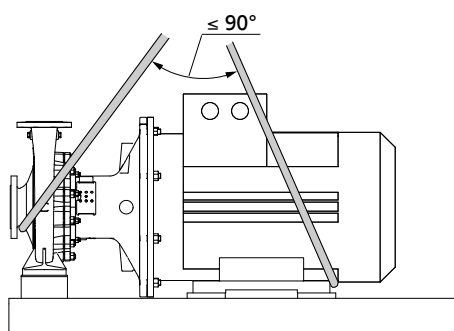
Рис. 3: Транспортировка насосного агрегата на фундаментной плите
